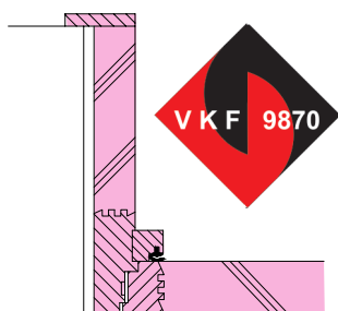
Abb.1 Normale Ausführung
