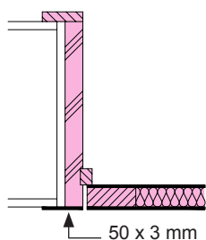
B Flacheisenrahmen
